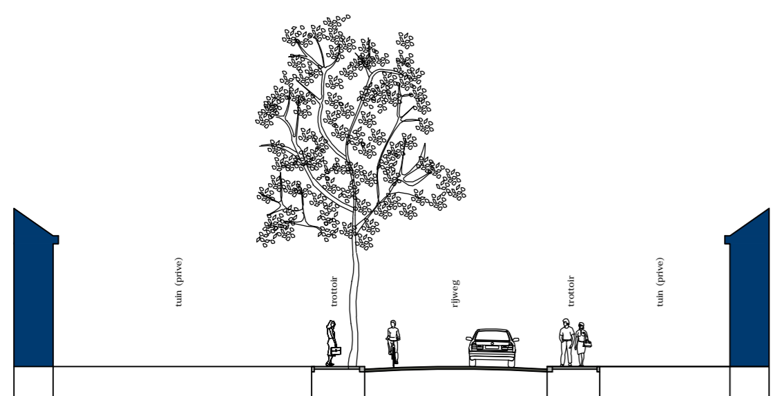
NORMAALPROFIEL MERGELAKKER Bestaande situatie
