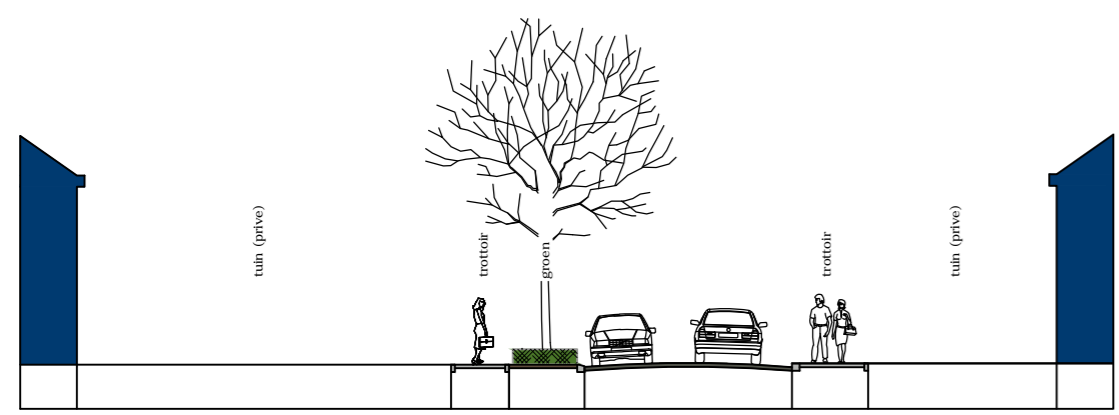
NORMAALPROFIEL MERGELAKKER Nieuwe situatie
